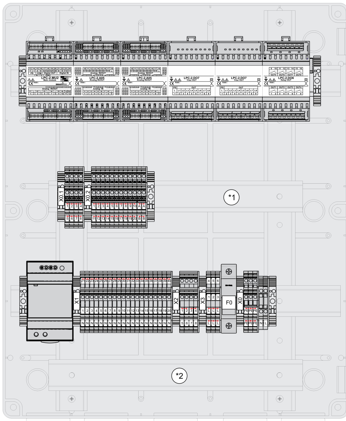
Slika 4: SHC-002 znotraj
