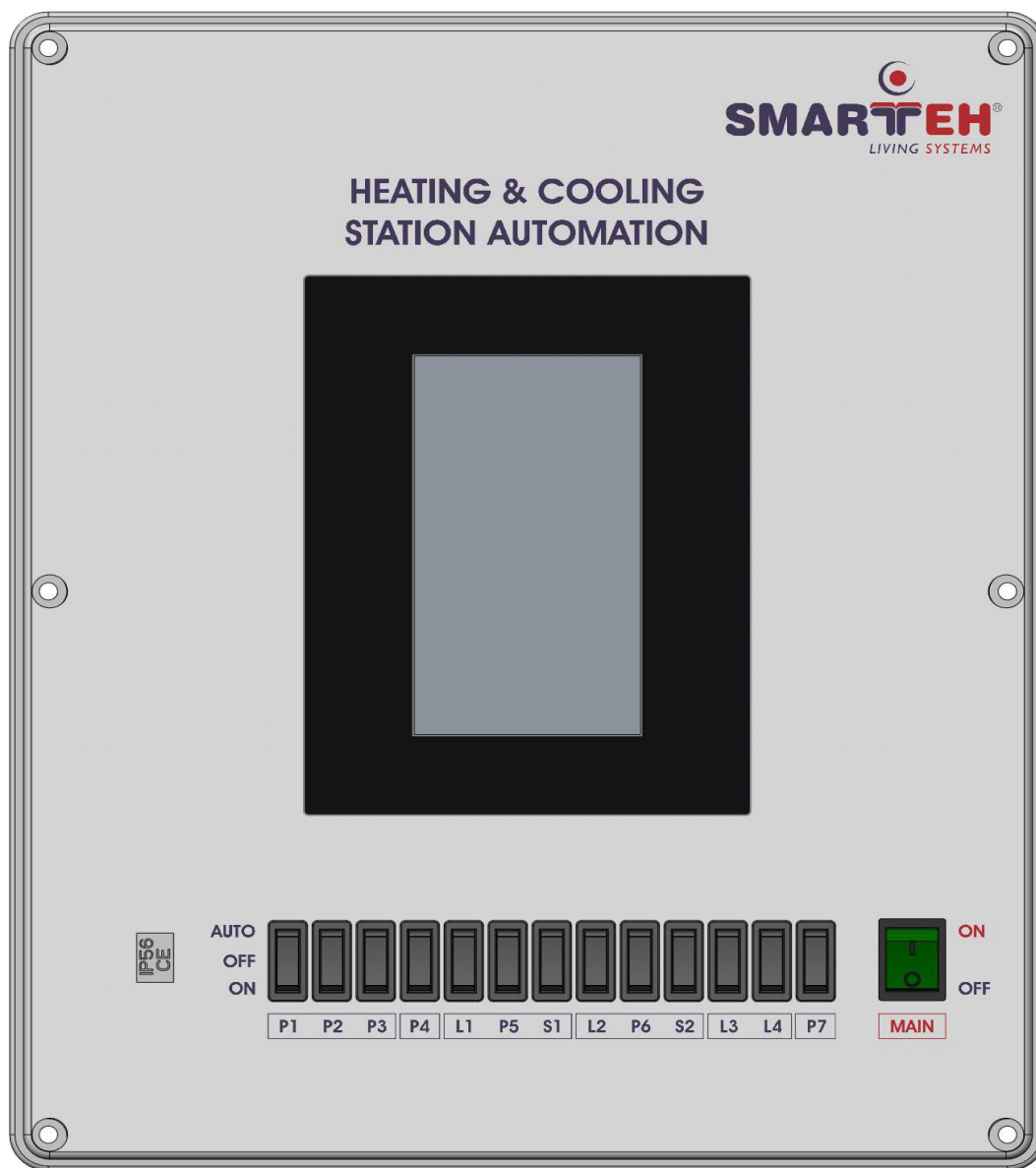
Slika 3: SHC-002
