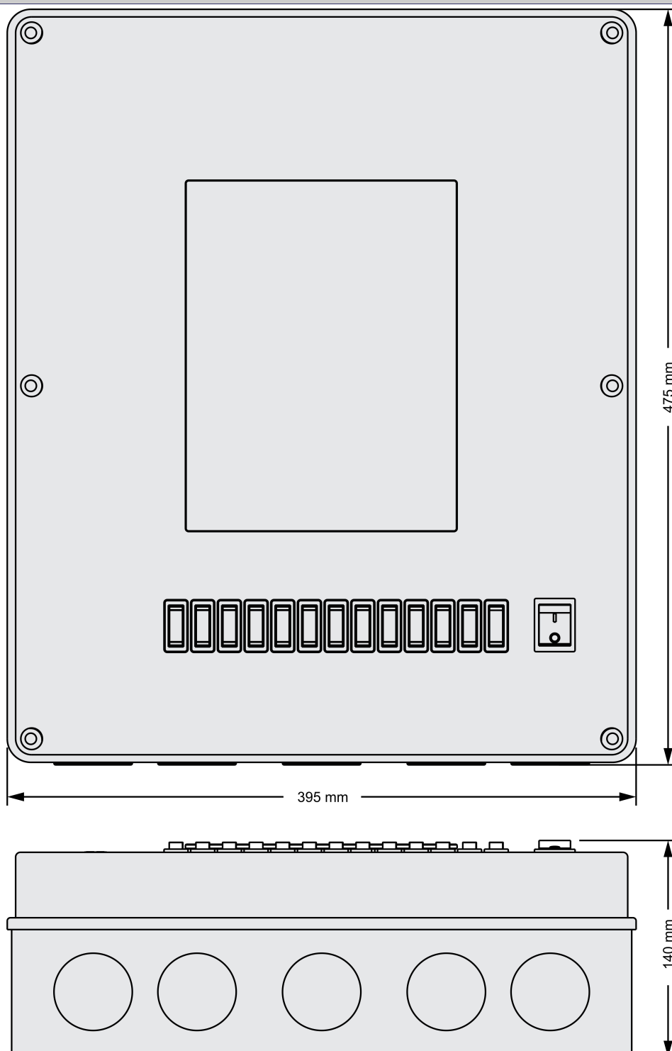
Slika 7: Dimenzije ohišja
