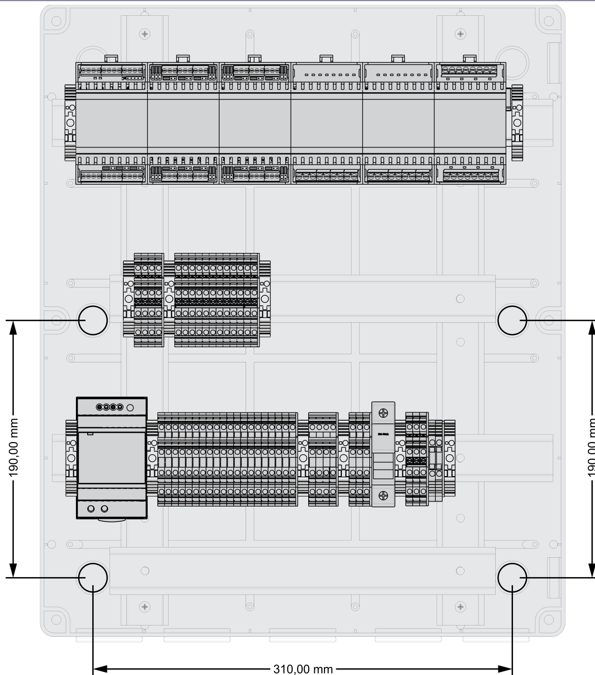
Slika 8: Položaj montažnih lukenj
