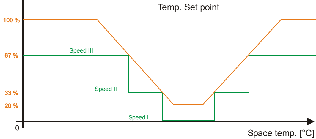
Fan reference output
